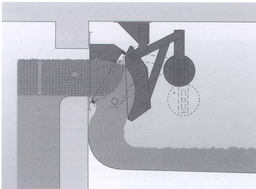
Funktionsbillede af RÜ afløbsklap
